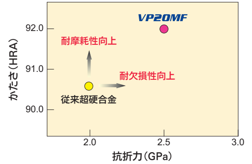
VP20MFの材料特性
