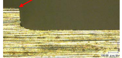
【超硬刀头扩大照片】
