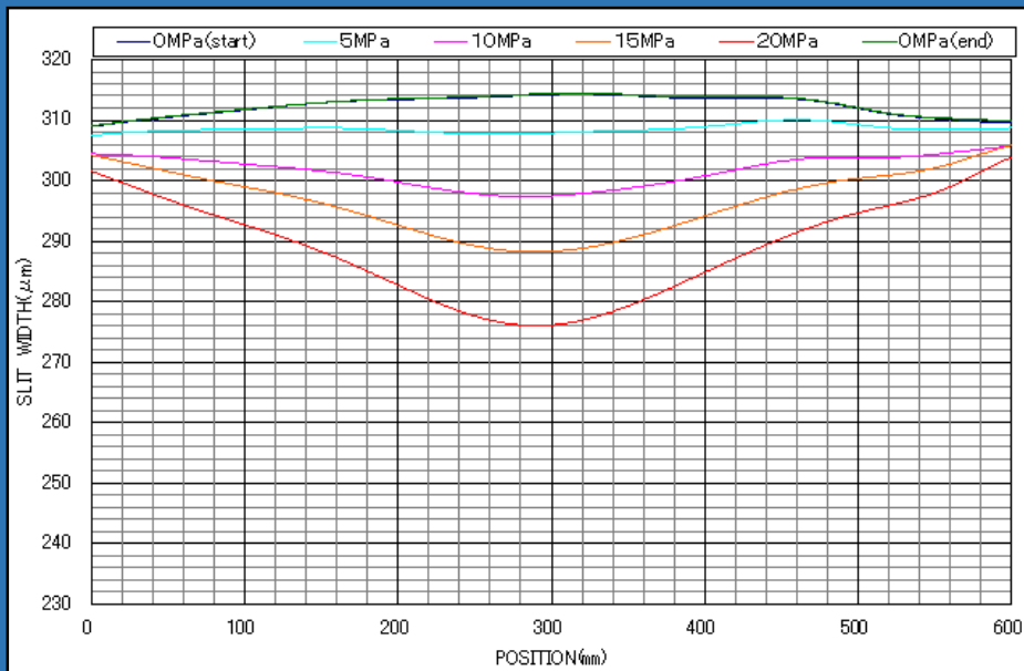
在600mm喷枪的中央设置一个液压组件
